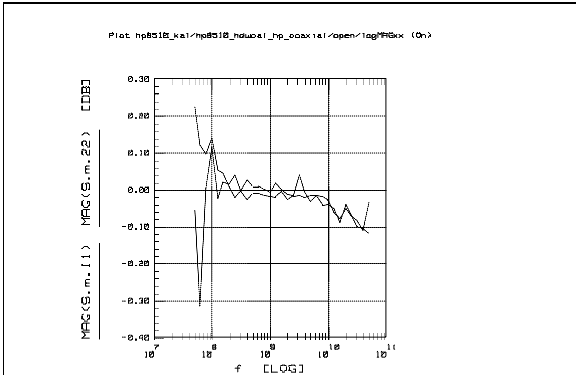
Bild 1: Variante A, logMAG(S11, S22) in dB für OPEN
