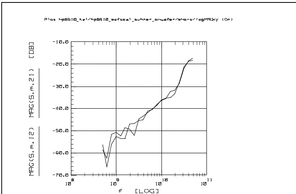
Bild 24: Variante E, logMAG(S21, S21) in dB für SHORT
