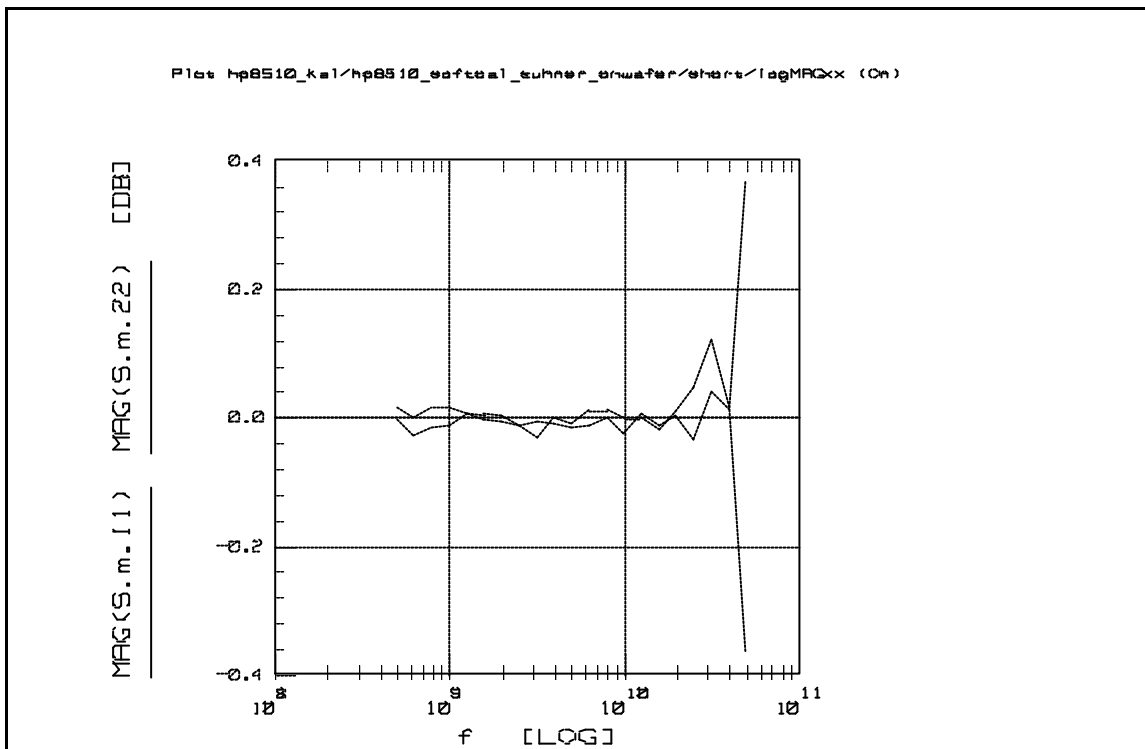
Bild 23: Variante E , logMAG(S11, S22) in dB für SHORT
